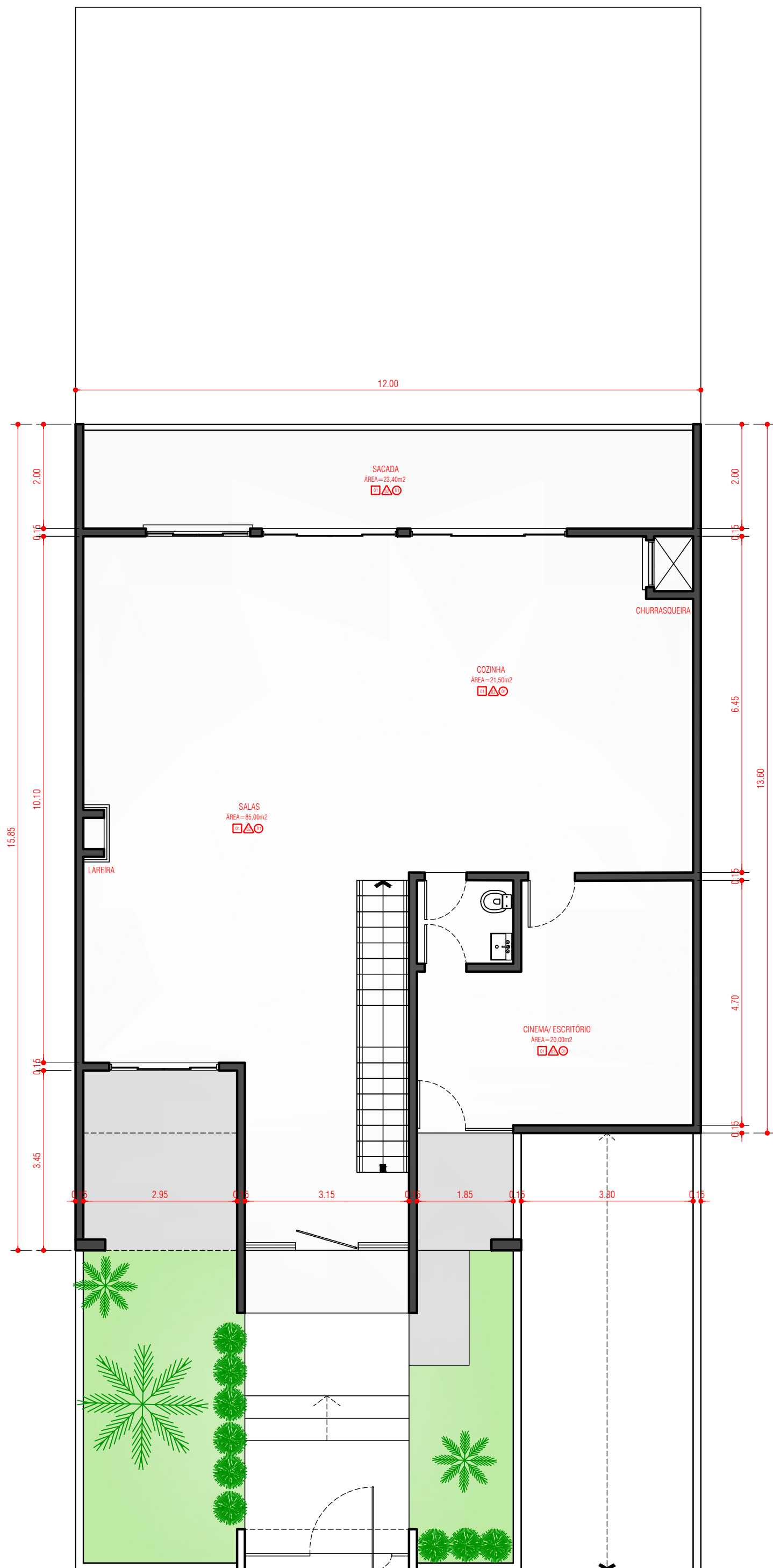
PLANTA BAIXA TÉRREO ÁREA PAVIMENTO = 182,10 m 2 ÁREA TOTAL = 688,93 m 2
