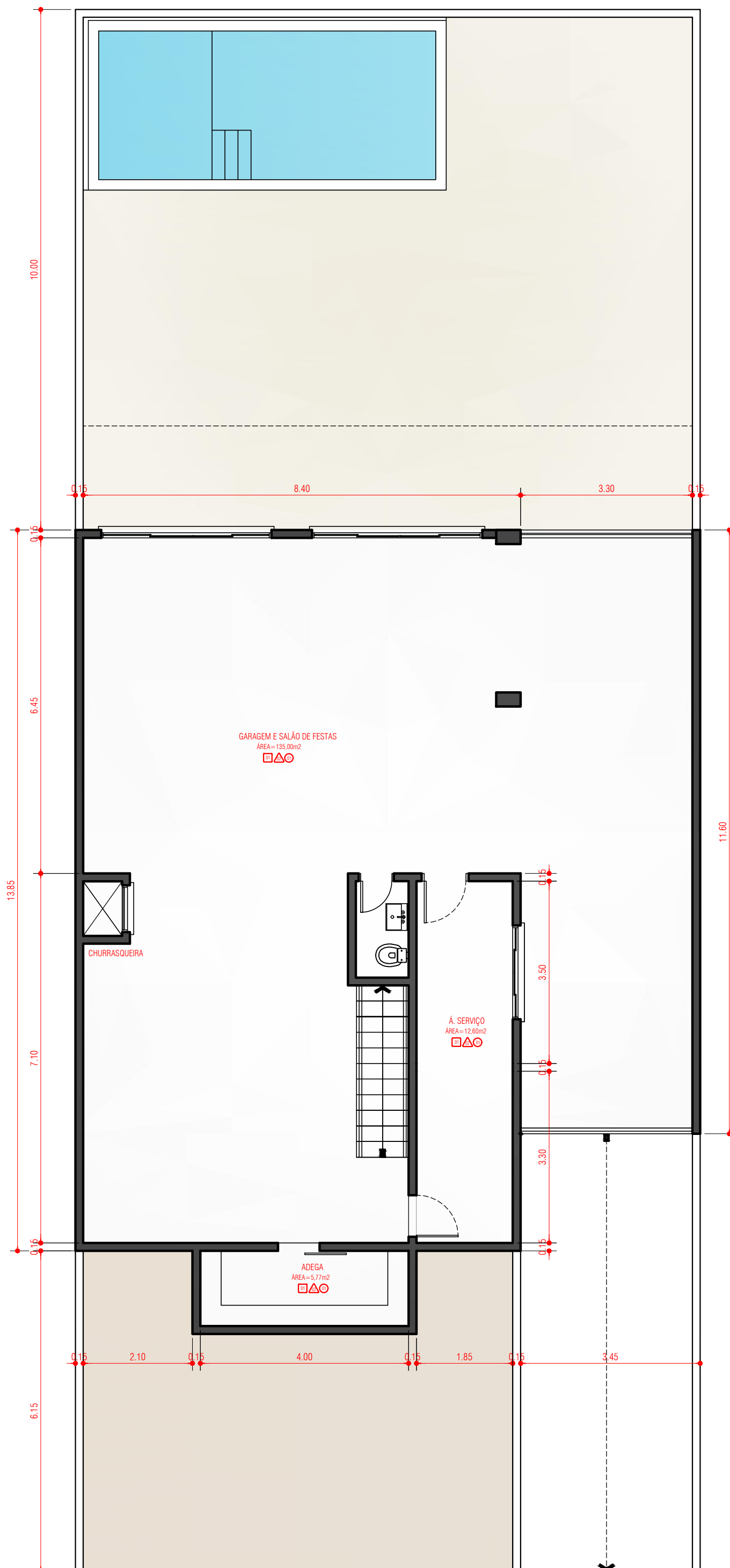
PLANTA BAIXA INFERIOR ÁREA PAVIMENTO=165,36 m2 ÁREA TOTAL=688,93 m2
